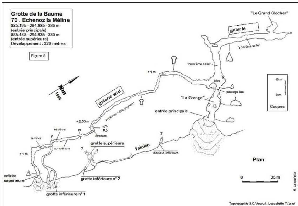
Figure 6 : Topographie de la Baume d'Echenoz. Spéléo Club de Vesoul
