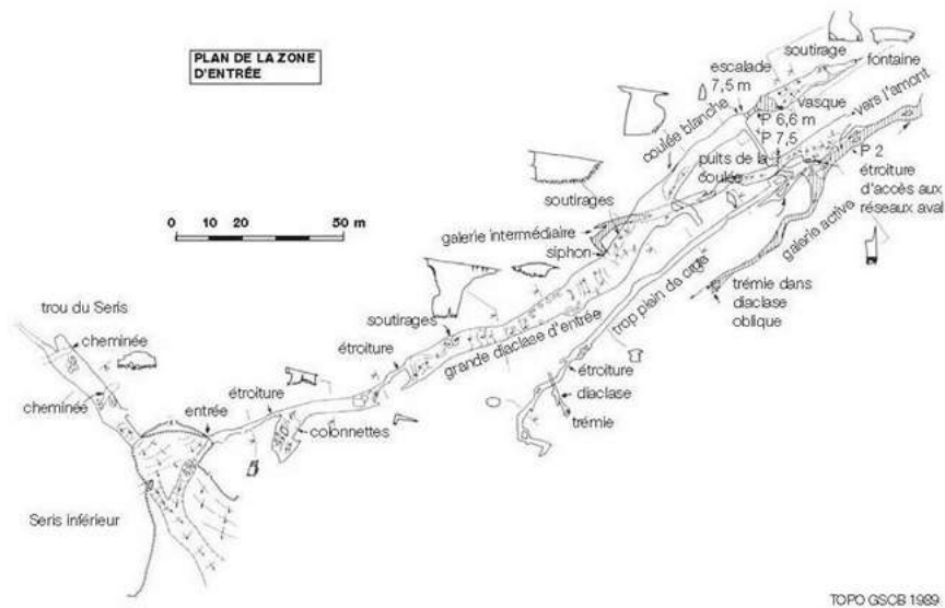
Figure 14 : Topographie de la rivière souterraine du Seris. Association Spéléologique du Doubs Central
