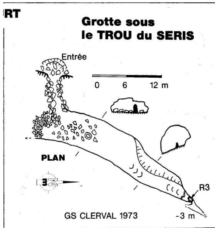
Figure 18 : Topographie de la grotte sous le Trou du Seris
