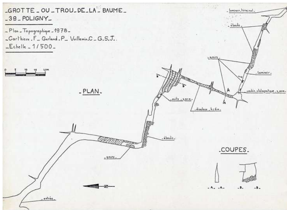
Figure 35 : Dernière topographie connue transmise par Christian Vuillemin. Il convient d'ajouter une centaine de mètres de développement après le laminar terminal élargi après 1978.
