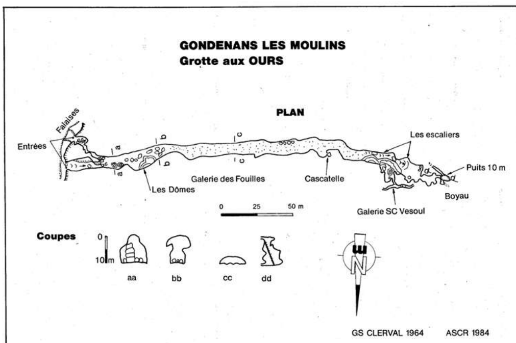
Figure 23 : Topographie de la grotte aux Ours de Gondenans
