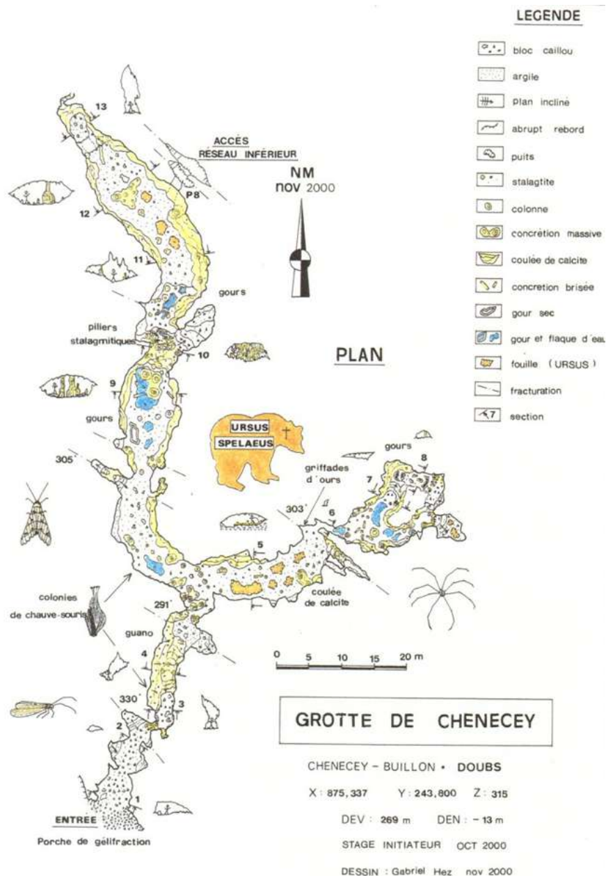
Figure 28 : Topographie de la grotte de l'Ours à Chenecey
