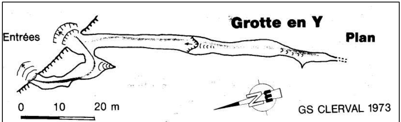
Figure 19 : Topographie de la grotte en Y
