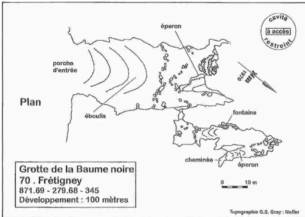
Figure 8 : Topographie de la Baume Noire. Groupe Spéléologique de Gray
