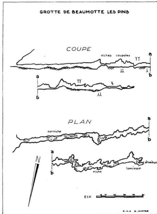
Figure 10 : Topographie de la grotte de Beaumotte-lès-Pins
