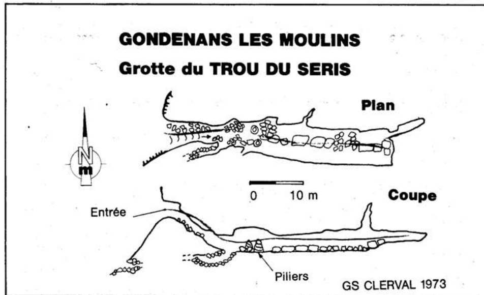
Figure 16 : Topographie de la grotte du trou du Seris. Association Spéléologique du Doubs Central
